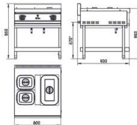
ЭМК-90/2П
