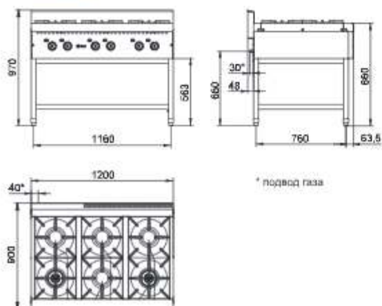
ПГК-69П
