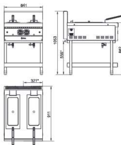
ГФК-90.2П
