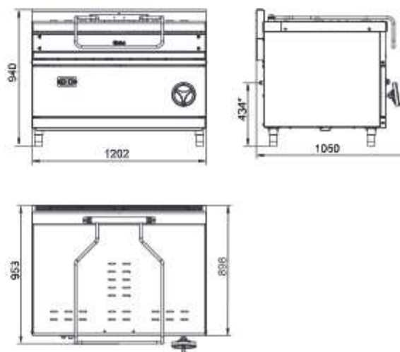
ГСК-90-0,67-150
