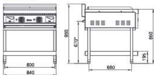
ГАКО-90П
