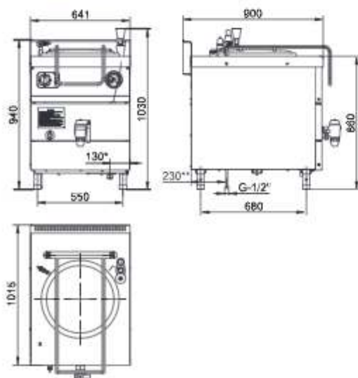
КРЕМ-60/9Т
