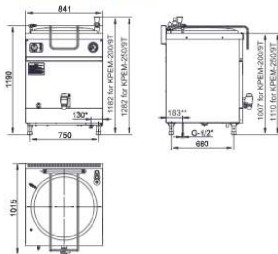
КРЕМ-200/9Т, КРЕМ-250/9Т
