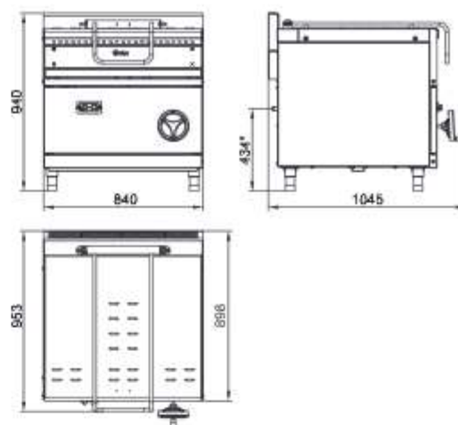
ГСК-90-0,27-40
