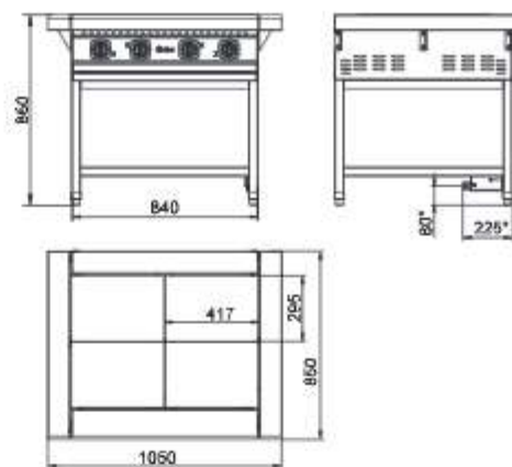
ЭП-4П
