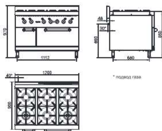
ПГК-69ЖШ
