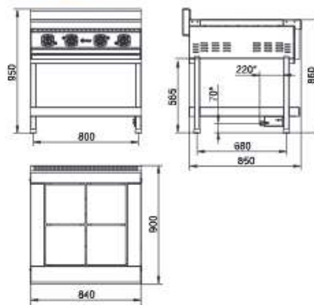
ЭПК-48П
