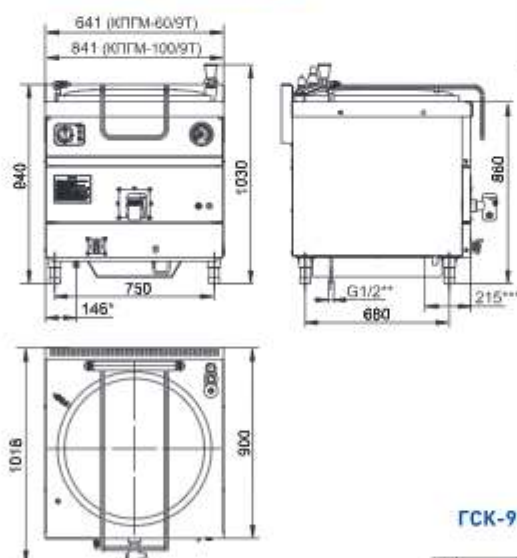
КПГМ-60/9Т, КПГМ-100/9Т
