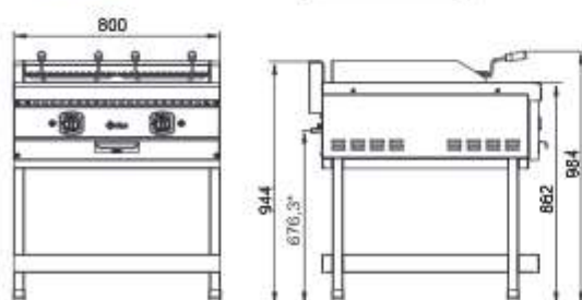
ГК-90П
