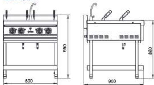
ЗБК-90/2П
