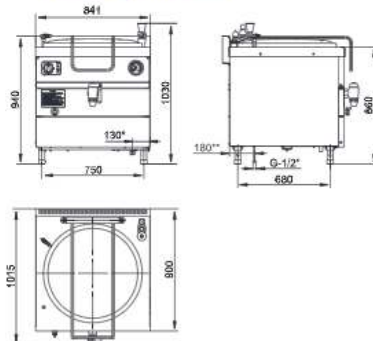
КПЭМ-100/9Т, КПЭМ-160/9Т
