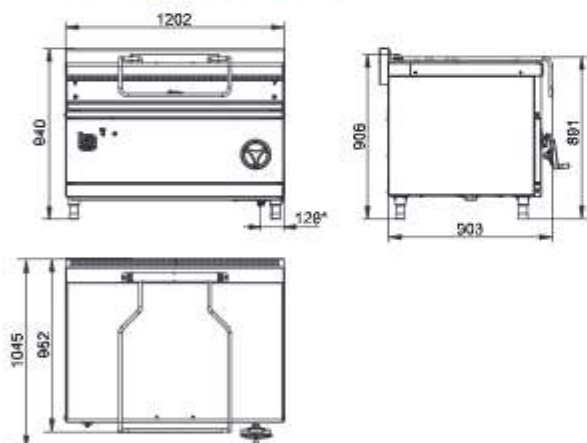
ЗСК-90-0,67-120, ЗСК-90-0,67-150
