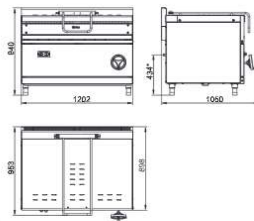
ГСК-90-0,67-120
