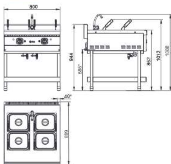
ГБК-90/2П
